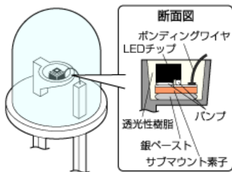
LEDランプ概念図
